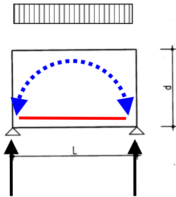
a) Appoggio diretto verticale: L'appoggio è costituito da punti d'appoggio sottostanti, la parete agisce come una trave su due o più appoggi
