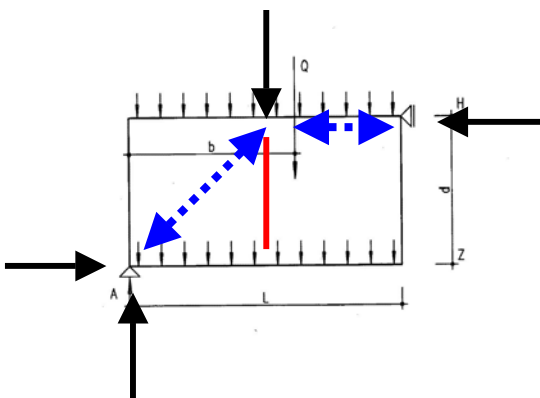
a) Appoggio diretto verticale: L'appoggio è costituito da punti d'appoggio sottostanti, la parete agisce come una trave su due o più appoggi
