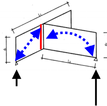
b) Appoggio indiretto verticale: L'appoggio a sinistra è costituito da una seconda trave parete che trasferisce le forze verticali fuori dal piano
